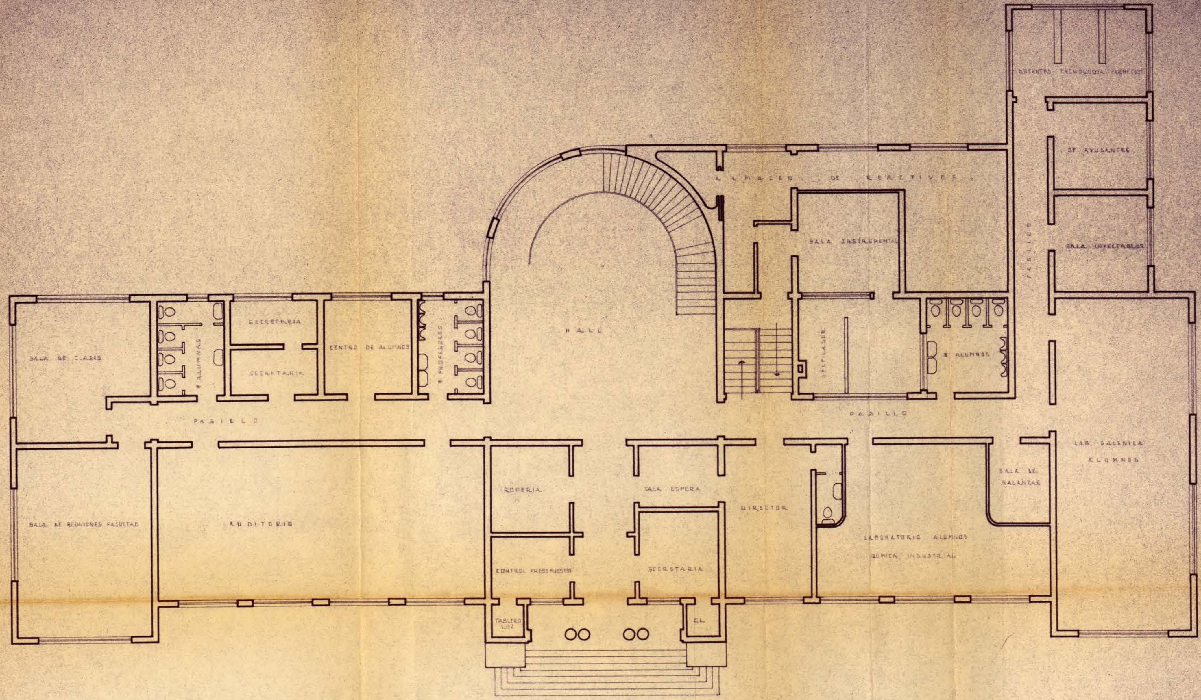
PLANTA PRIMER PISO Esc. 1:100
