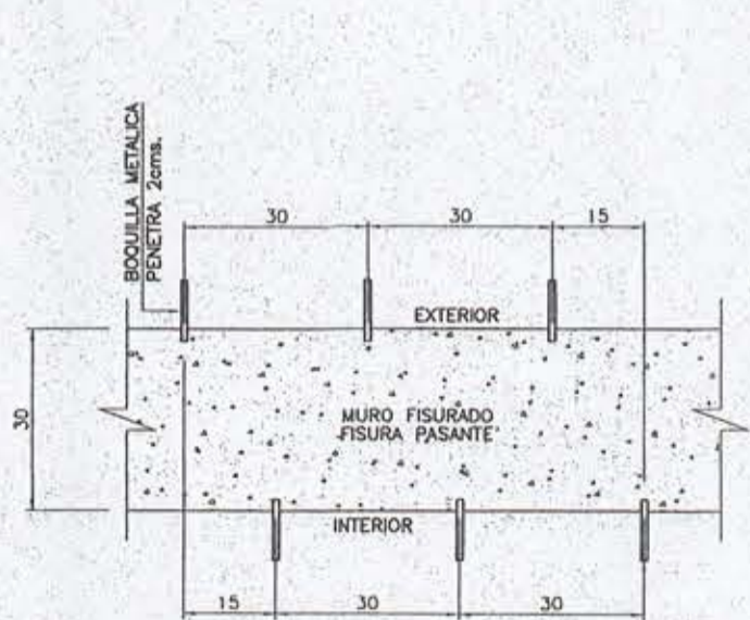
DETALLE COLOCACION (PLANTA) BOQUILLAS DE INYECCION ESC 1:10
