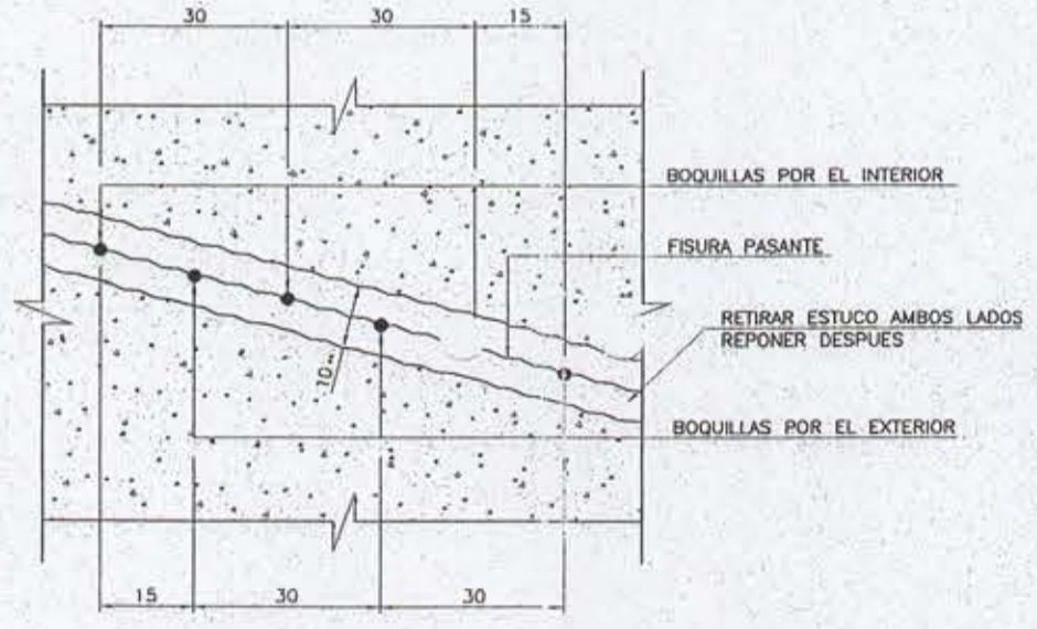
DETALLE COLOCACION (ELEV.) BOQUILLAS DE INYECCION ESC 1:10
