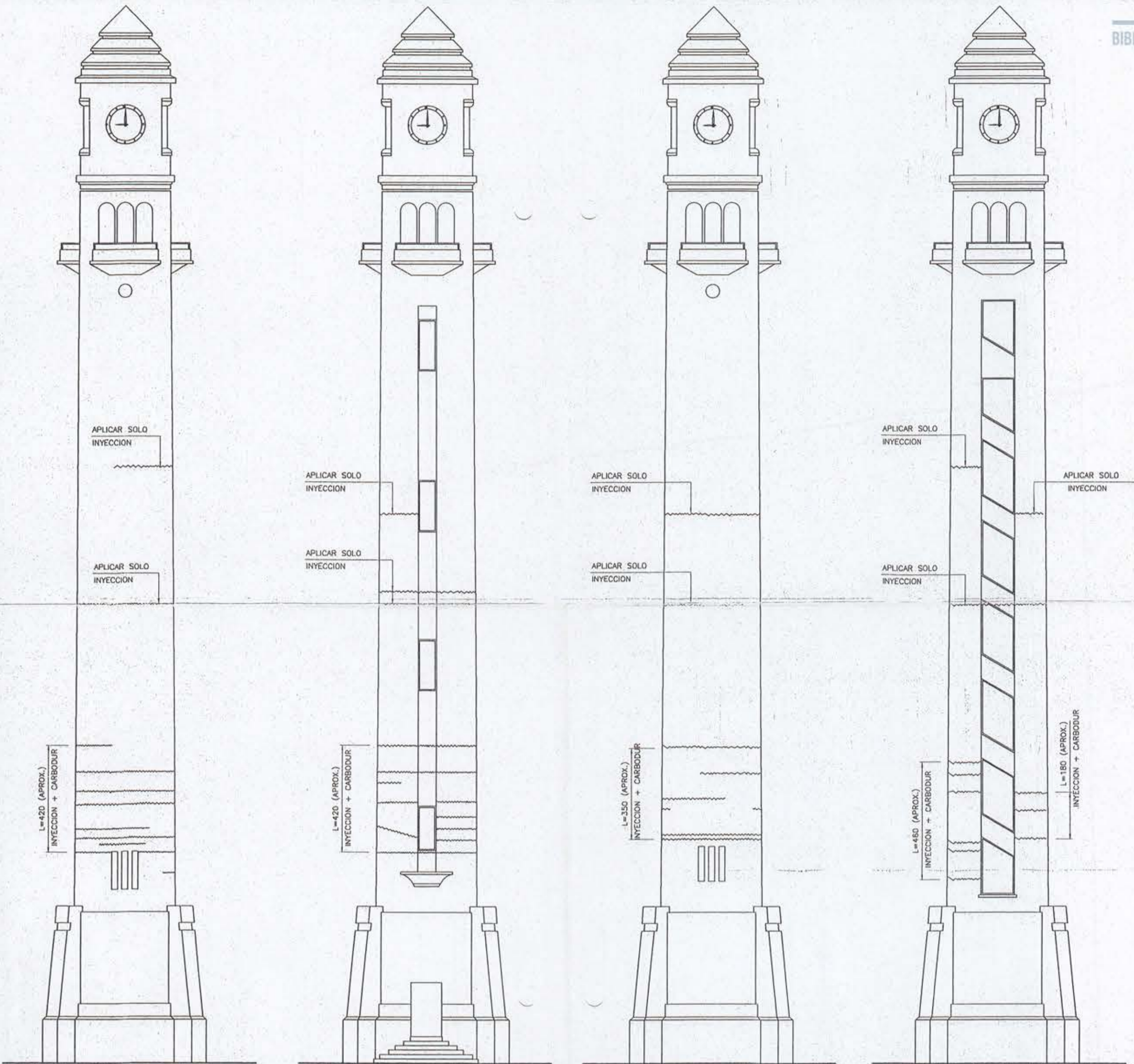
ELEVACION SUR ESC 1:100
