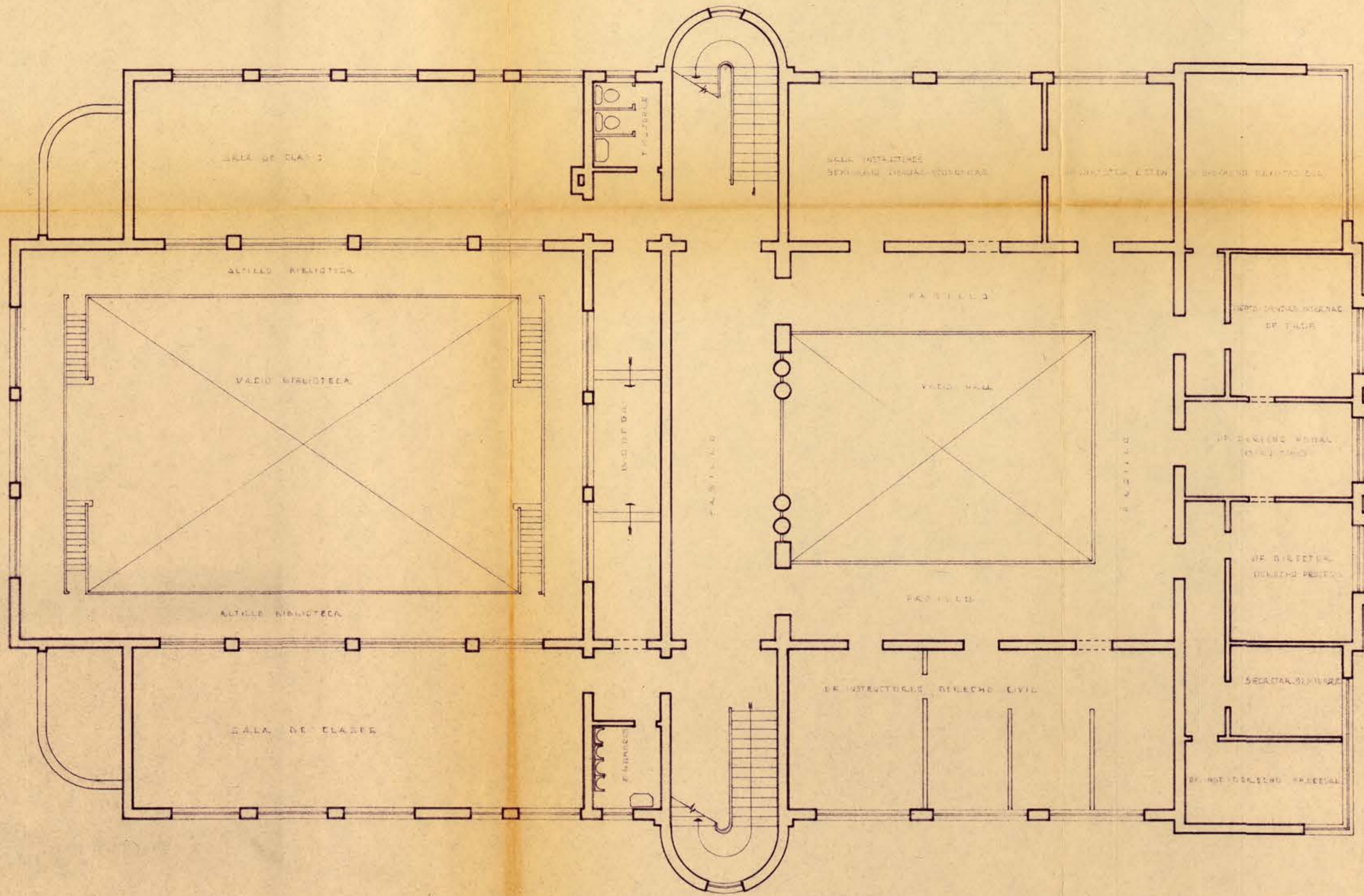
Planta tercer piso Esc.1:100
