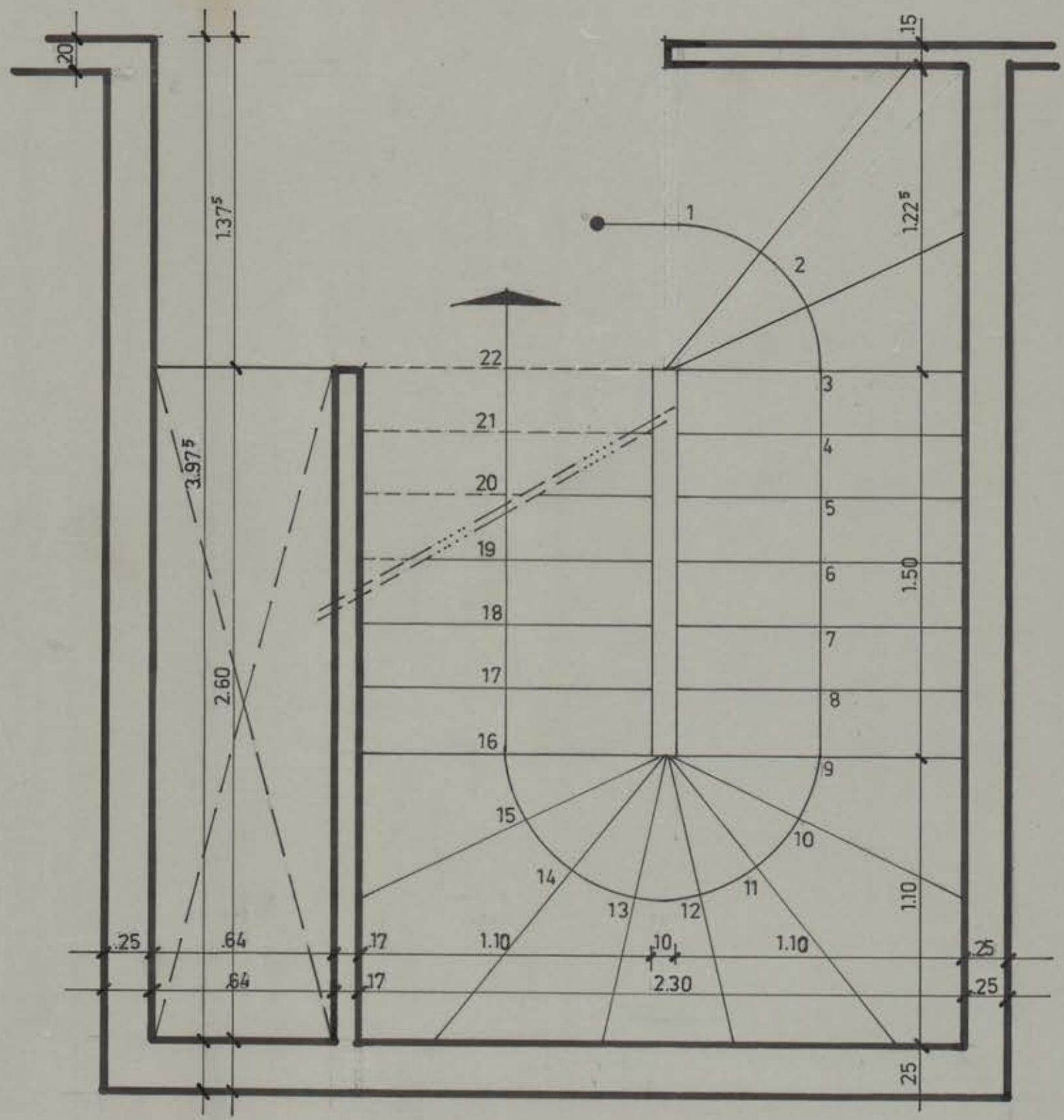
PLANO PLANTA ESCALERA N° 11 (de 1ª a 2ª pisos) E = 1:20
