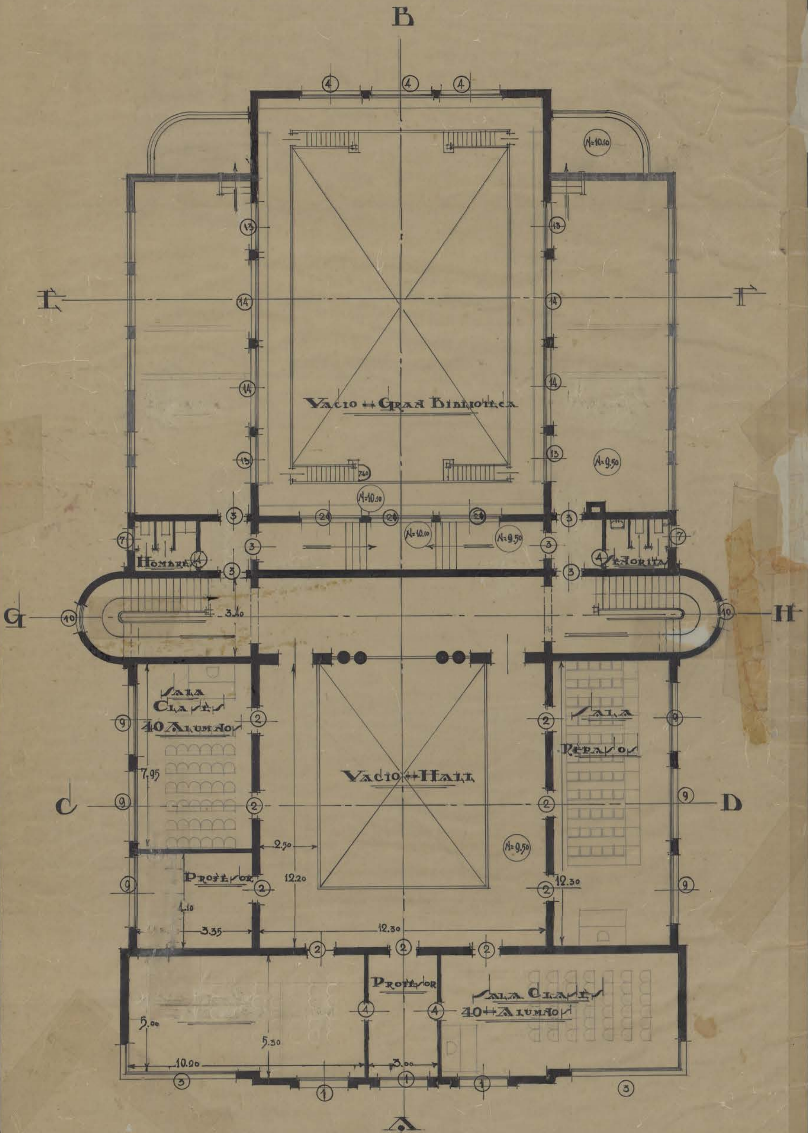
PLANO DEL TERCER PISO
