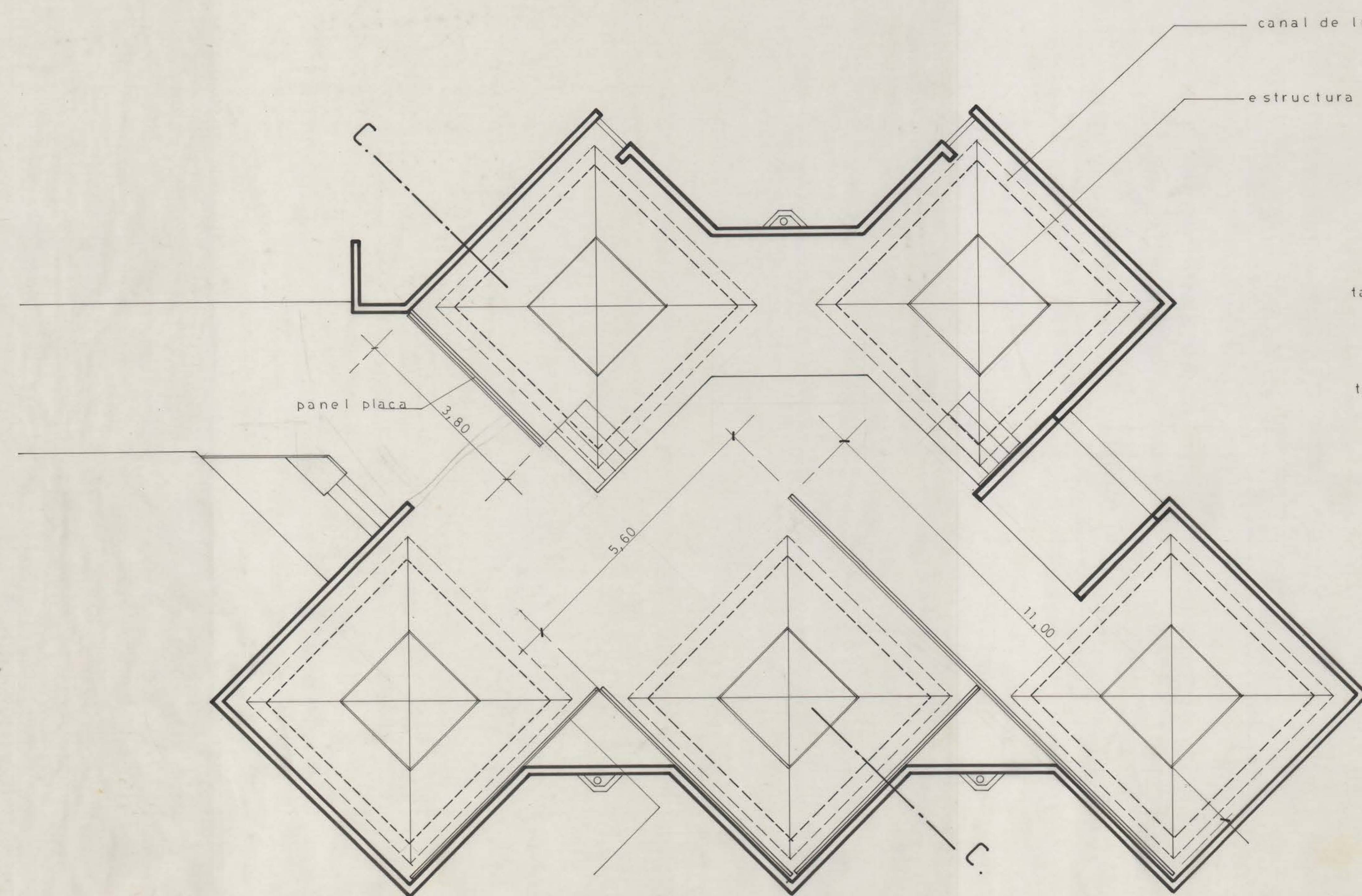
PLANTA CIELO LUMINOSO SALA DE EXPOSICION ESCALA 1:50.
