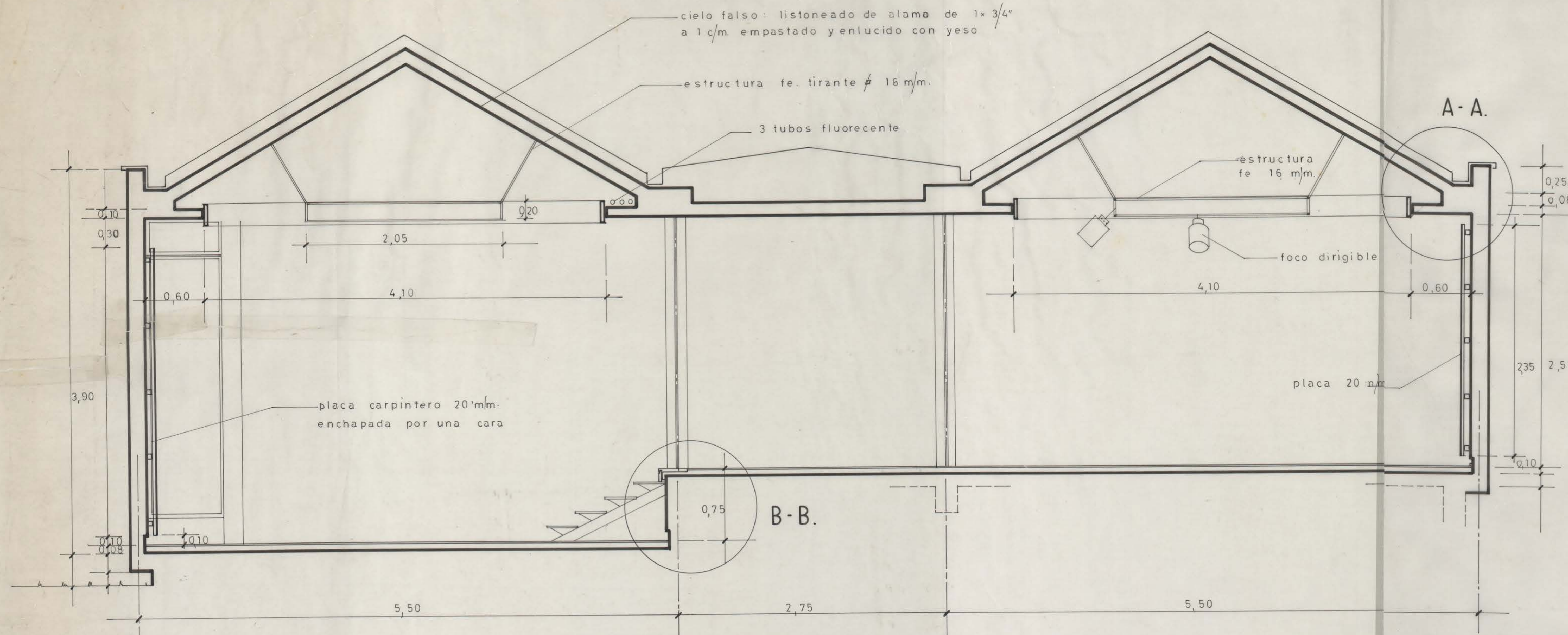
ELEVACION EN CORTE C-C. ESCALA 1:20
