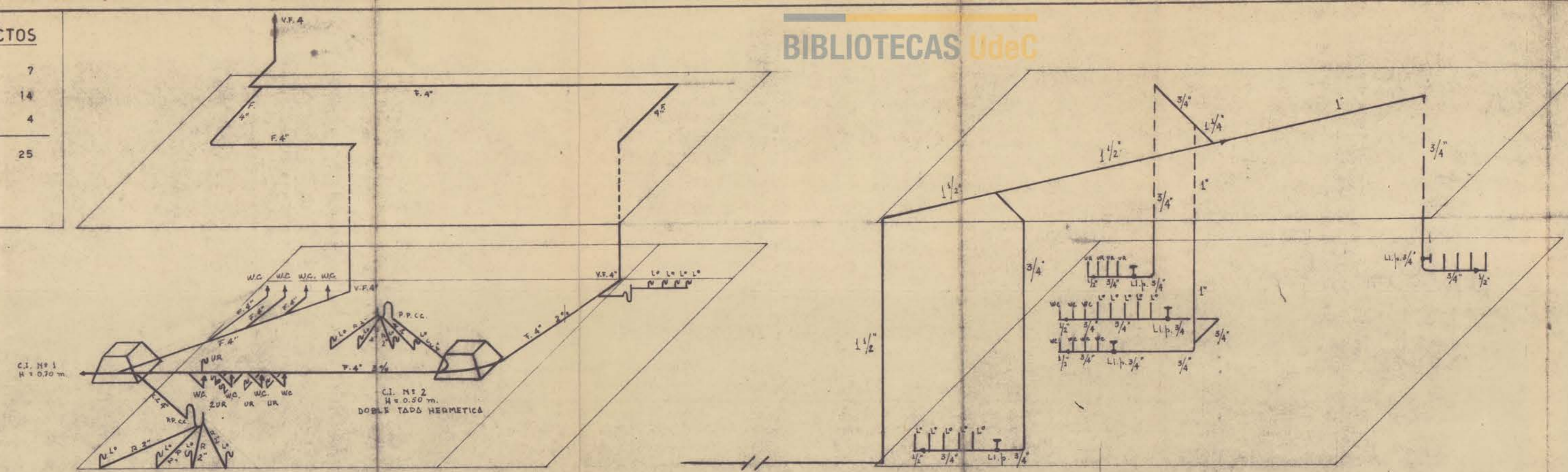
ESQUEMA ISOMETRICO DE AGUA POTABLE
