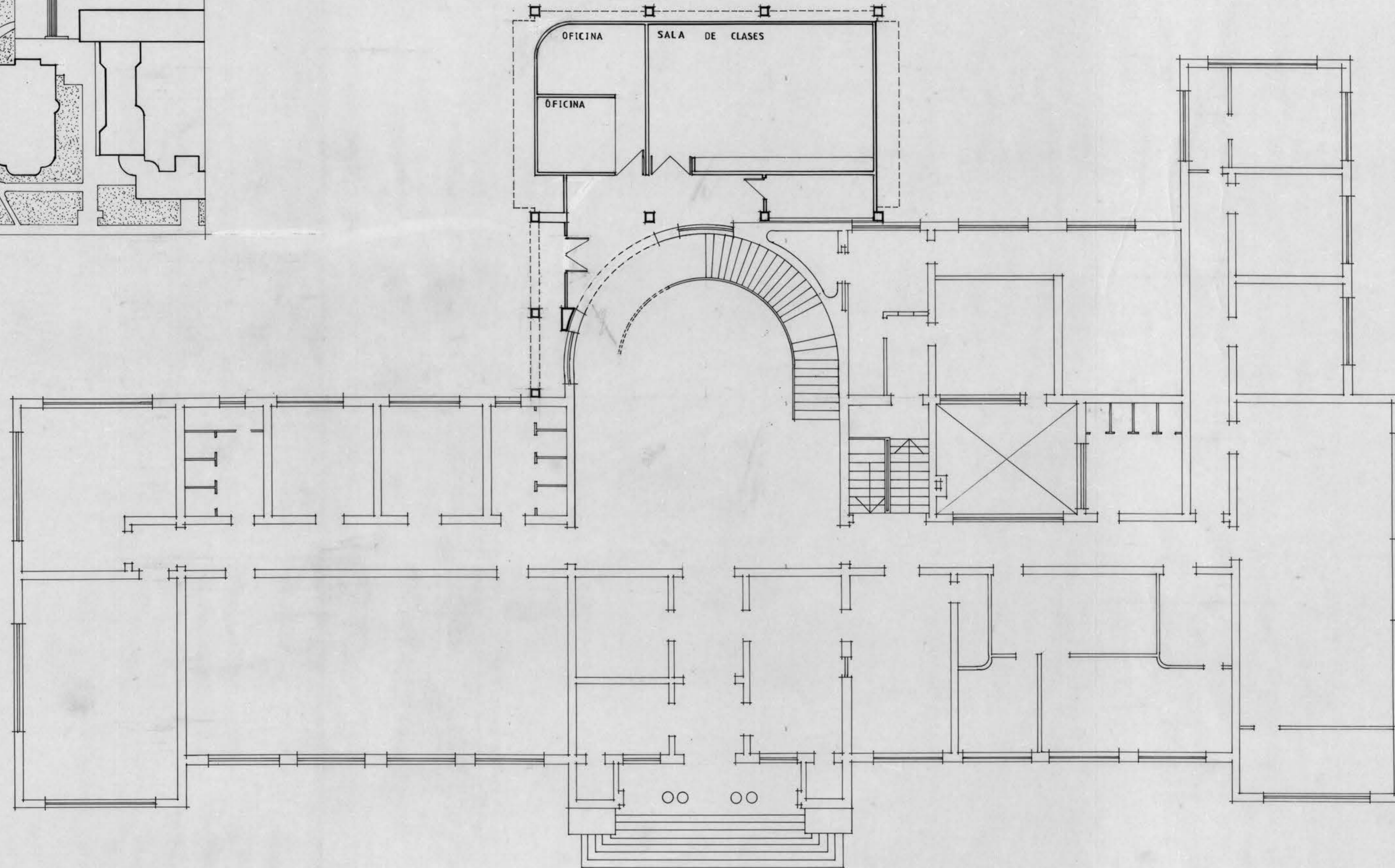
PLANTA 1º PISO ESCALA : 1 : 100
