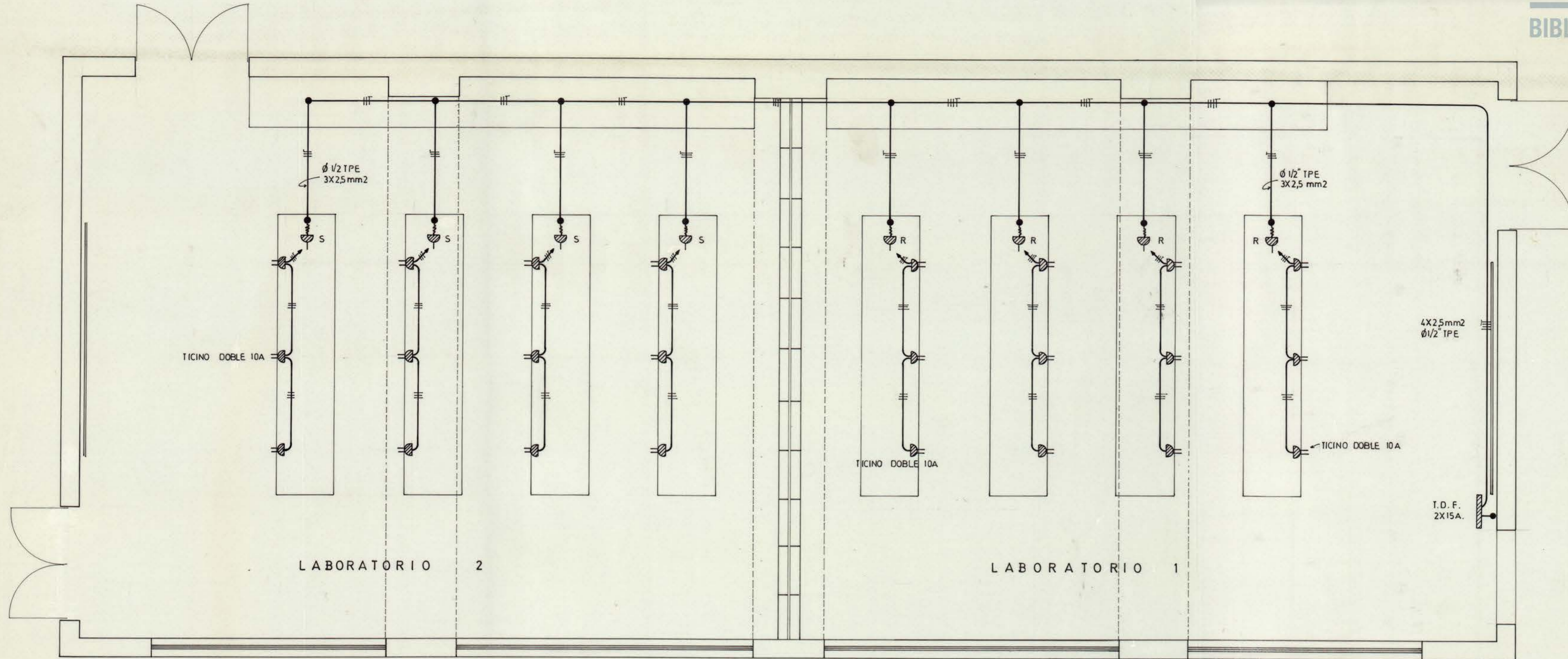
PLANTA ESC. 1:25
