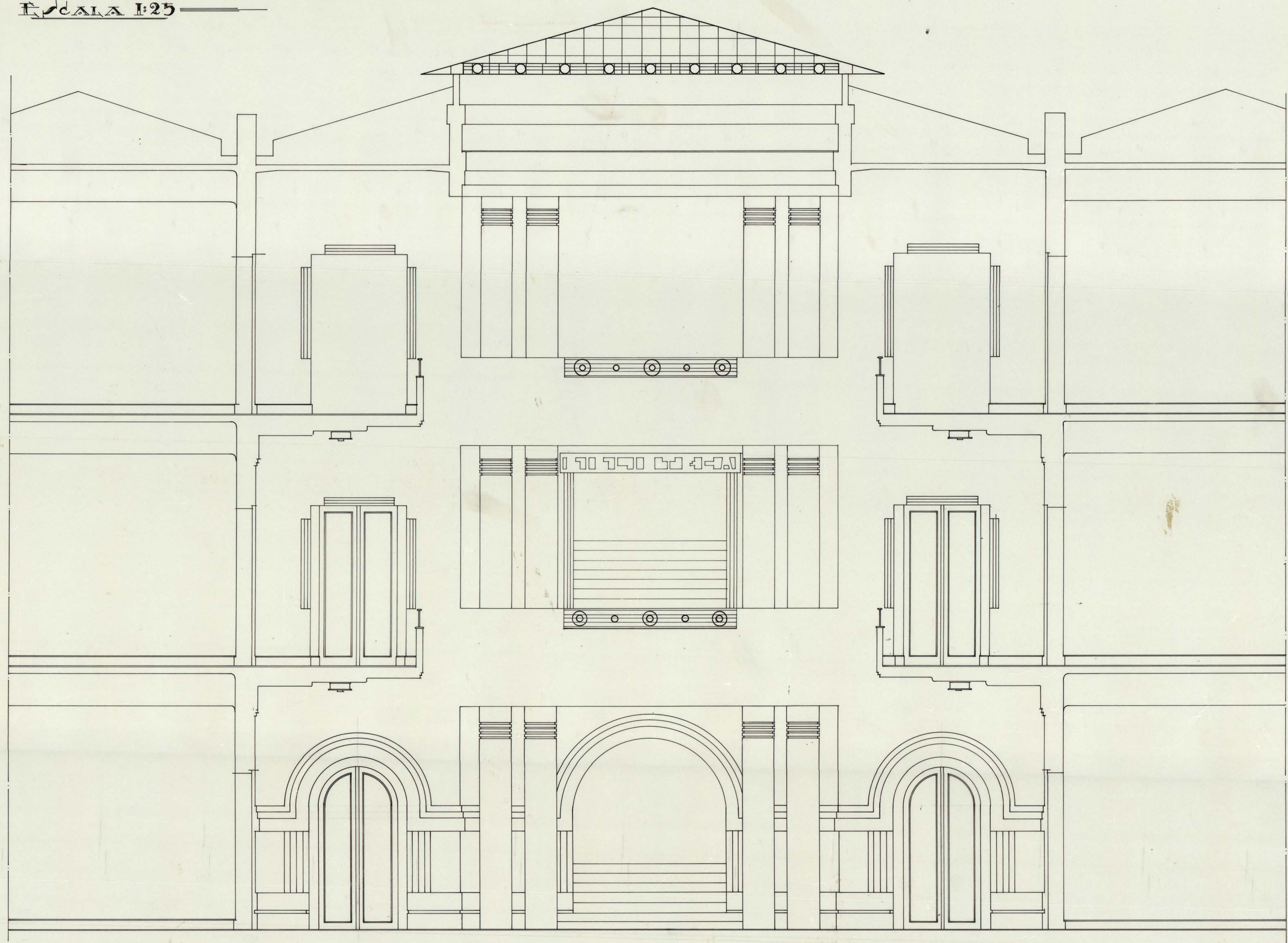
DETALLE DEL HALL EN SECCION TRANSVERSAL
