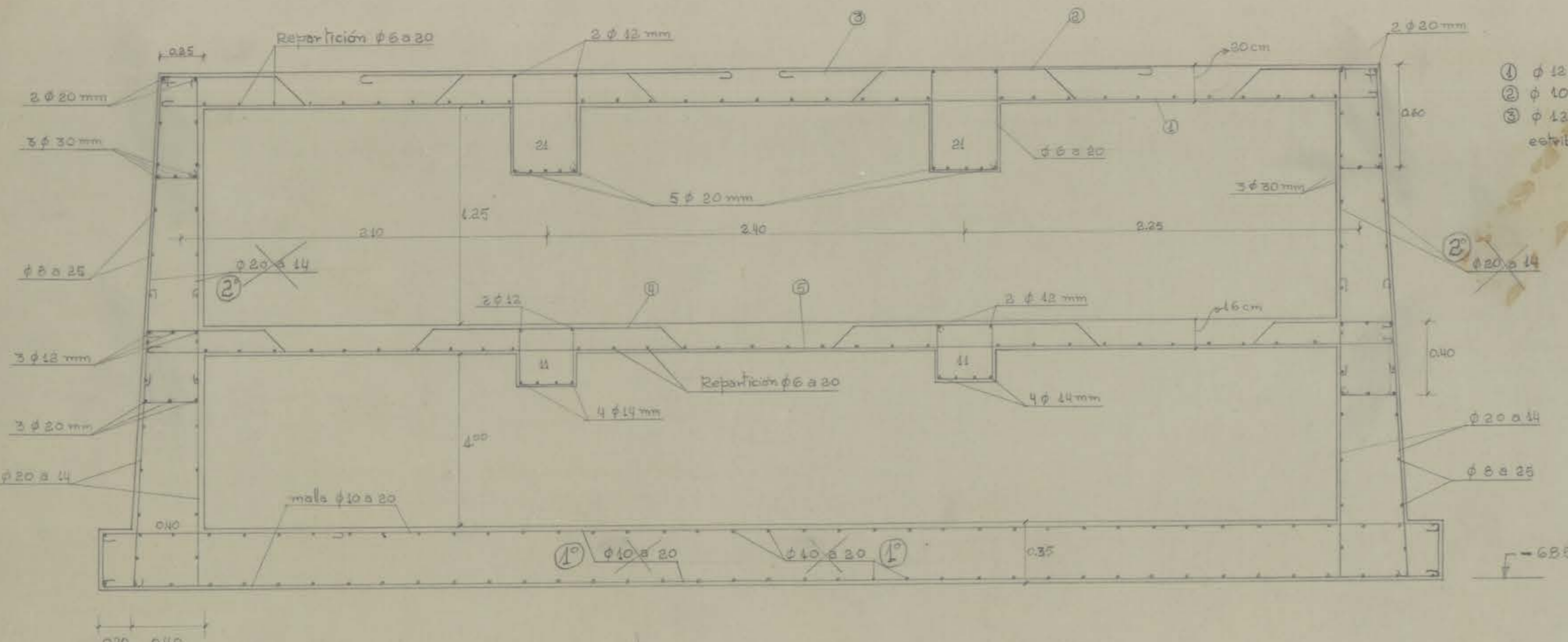
CORTE D-D ESC. 1:20
