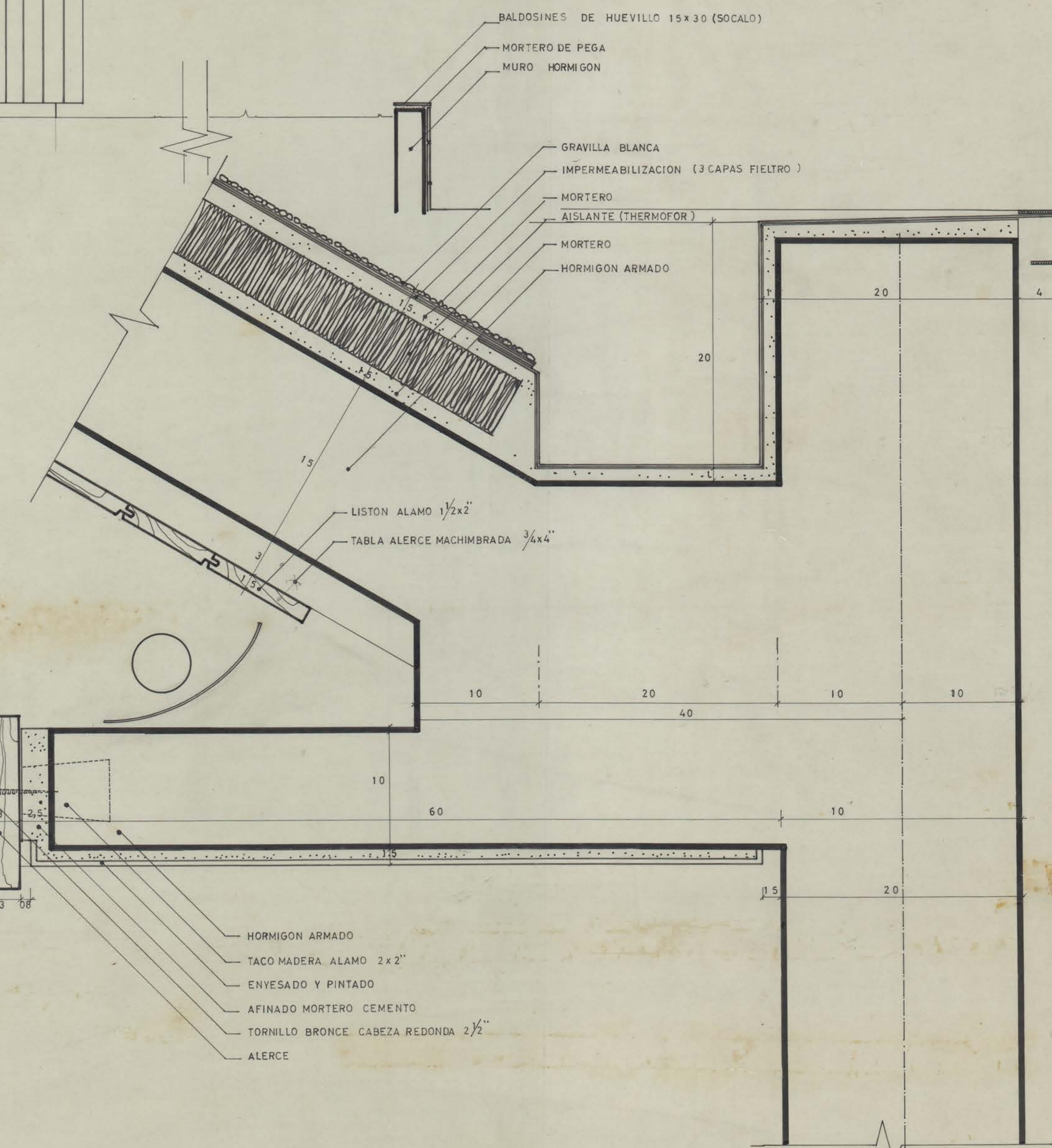
DETALLE CORTE C C
