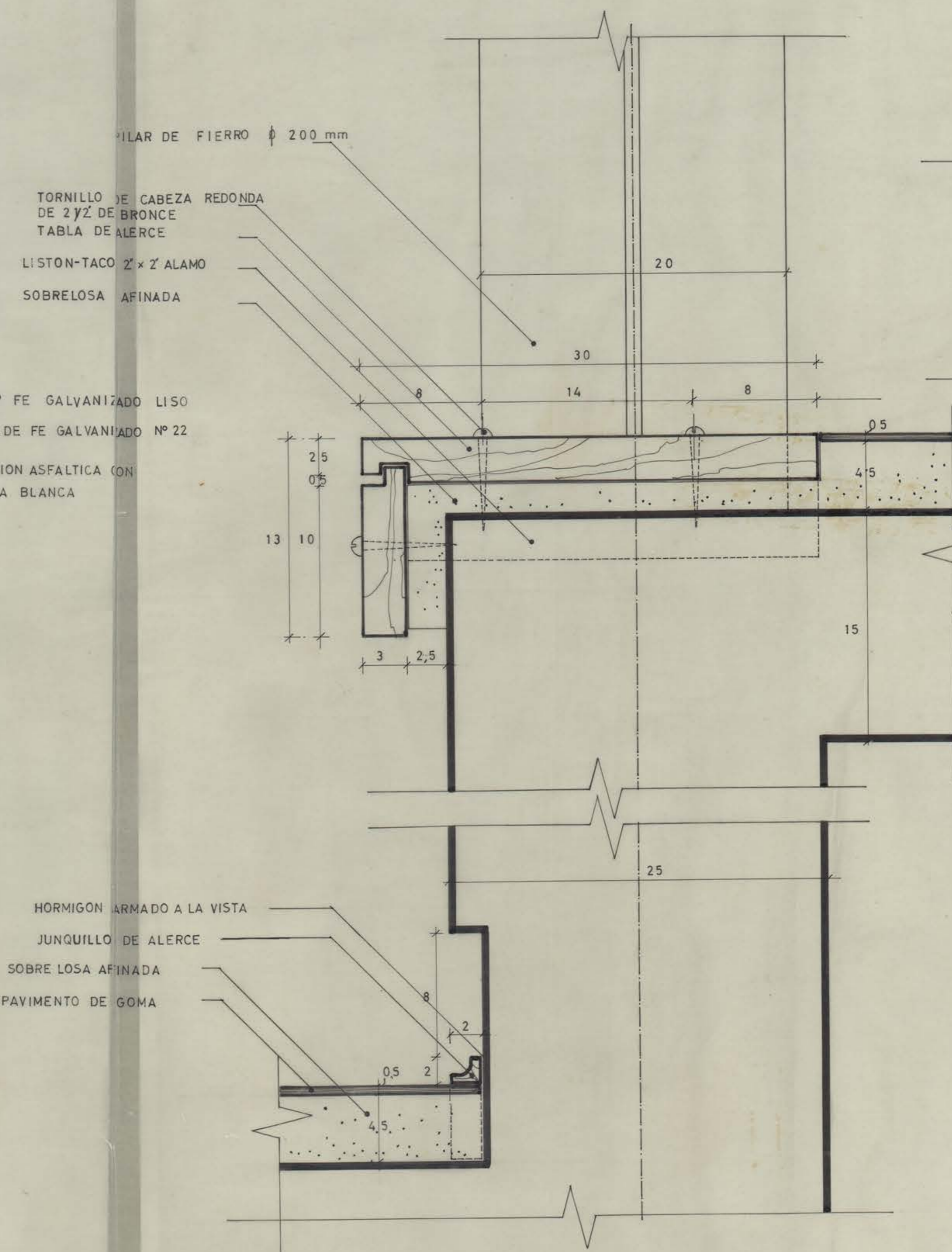
DETALLE CORTE AA
