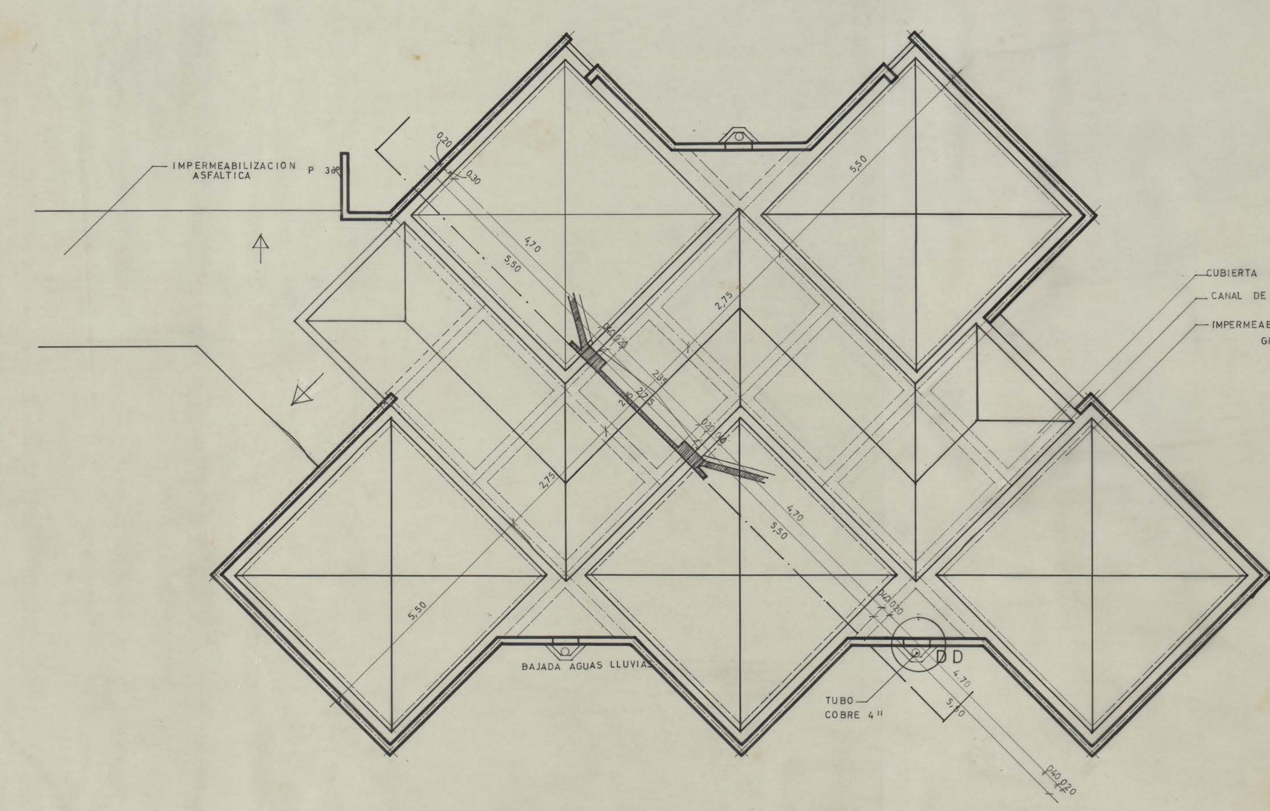
PLANTA DE TECHUMBRE
