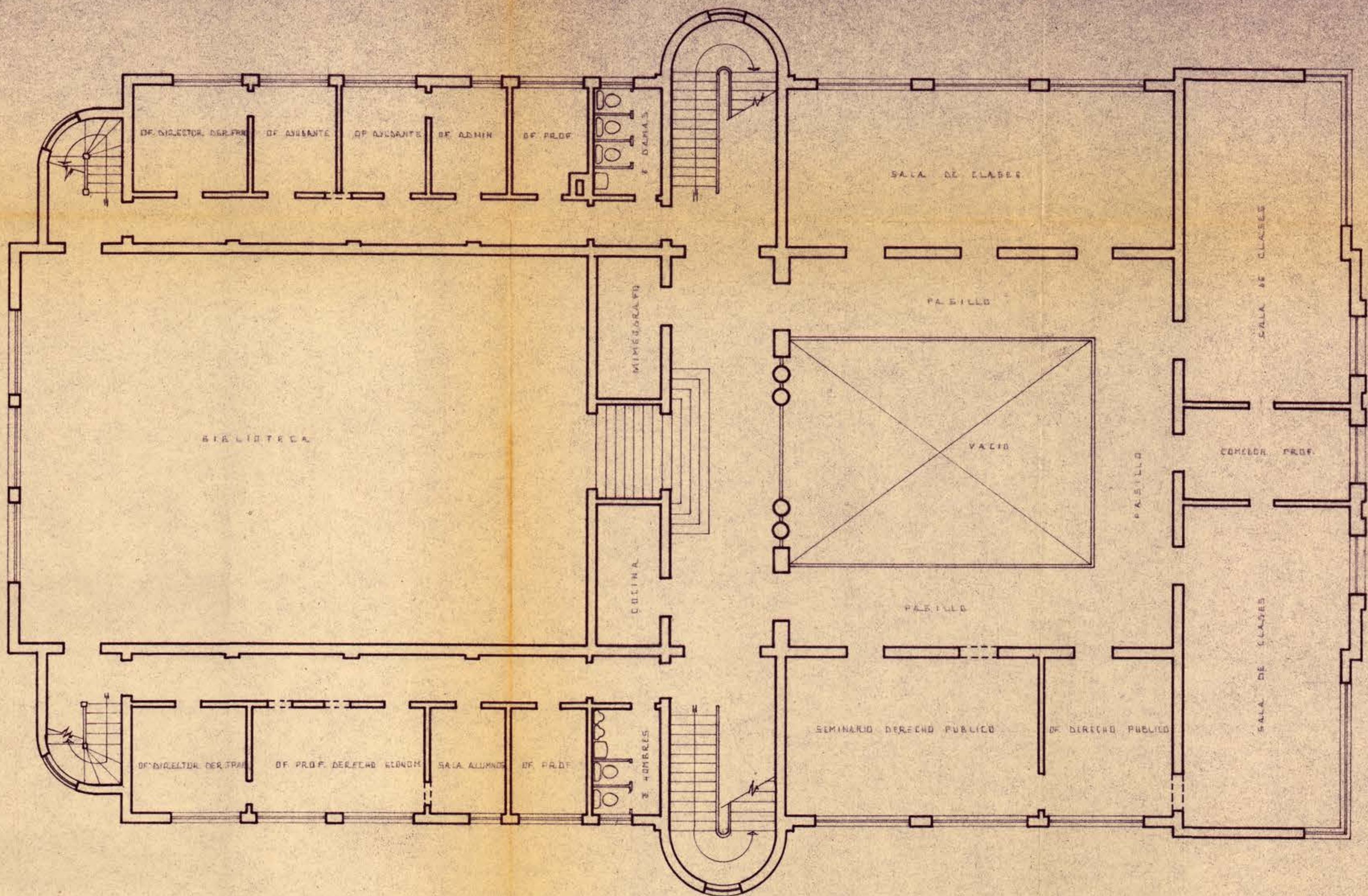
Planta segundo piso Esc. 1:100
