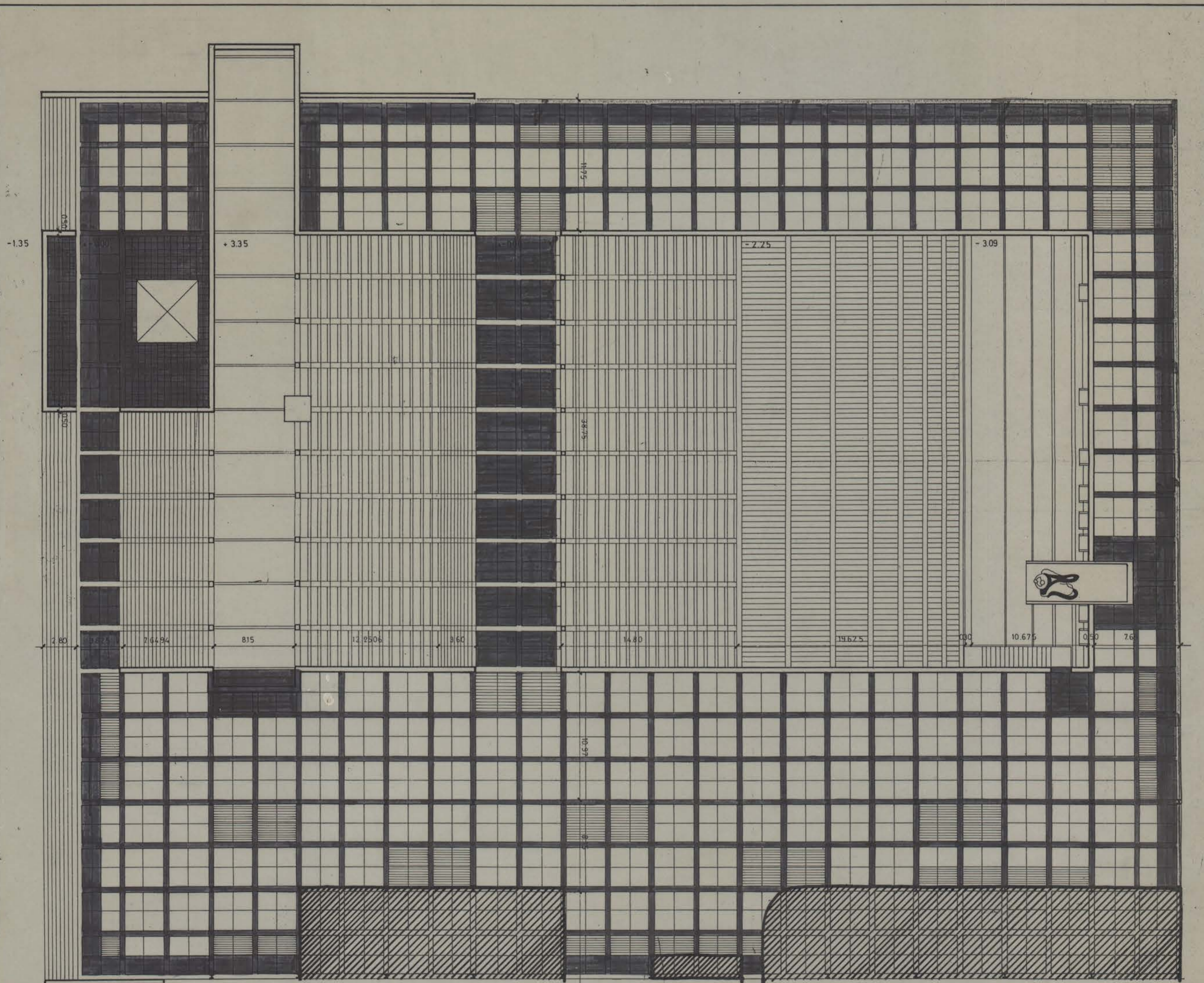
PLANTA PAVIMENTOS 1:200
