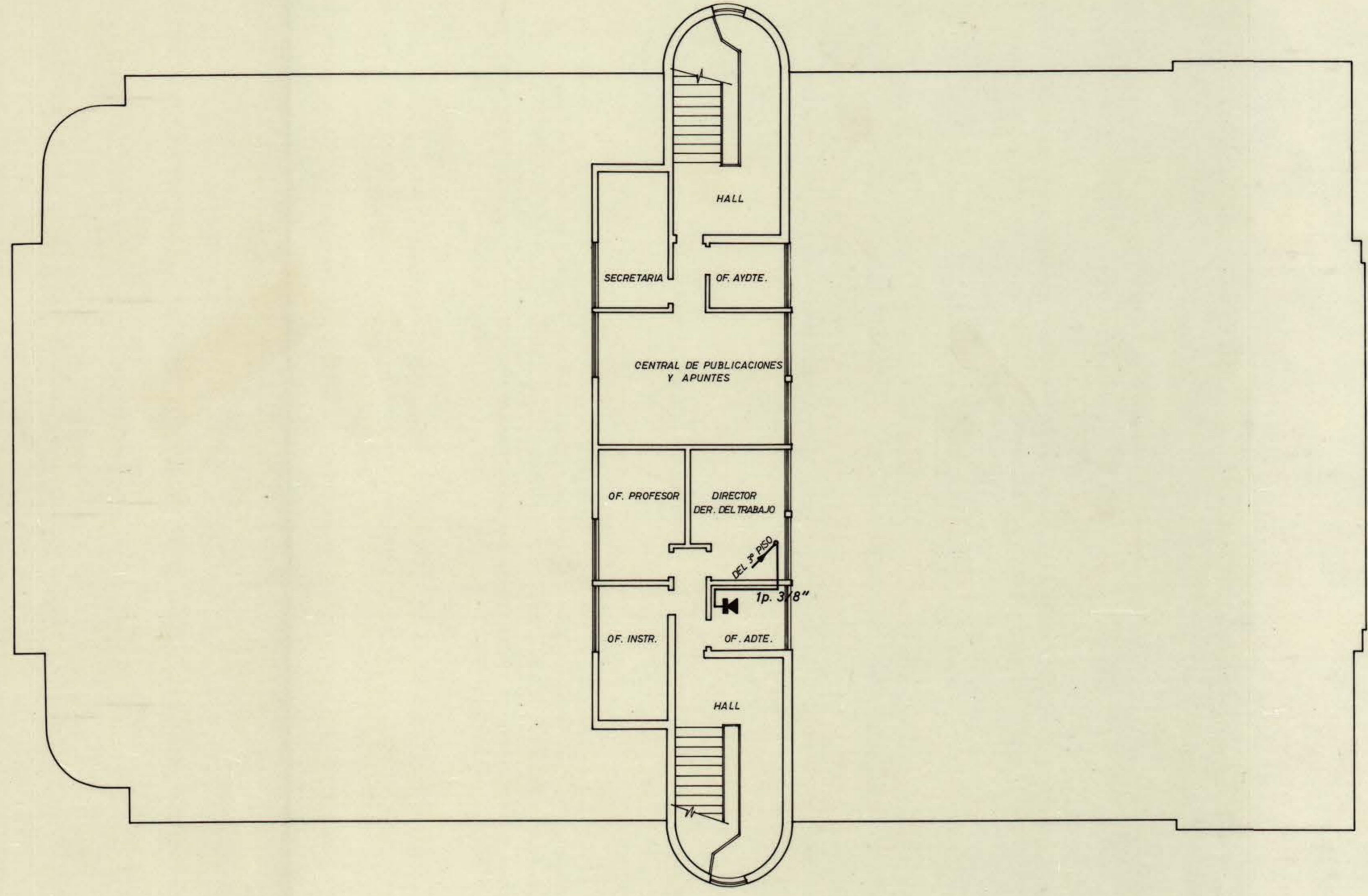
PLANTA DEL CUARTO PISO ESC. 1:100
