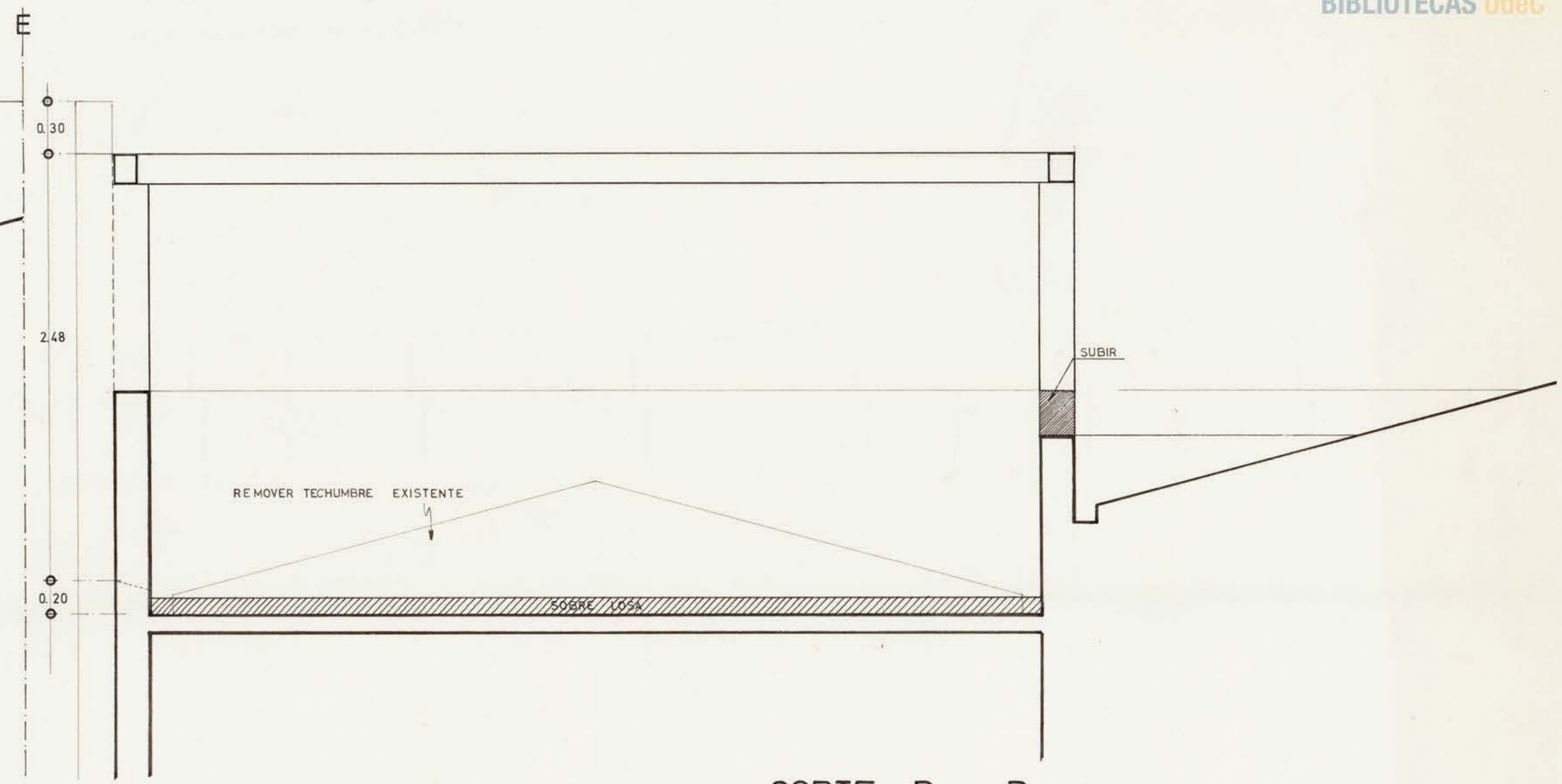
CORTE B-B
